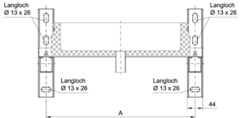
Montagemaße Wandmontage bei "Montageschiene" Typ 325 und Typ 475
