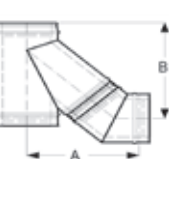
Abb. T-Stück 45° mit Bogen 45°
