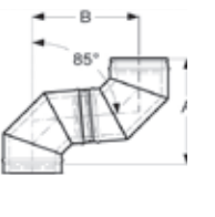
Abb. Bogen 85°
